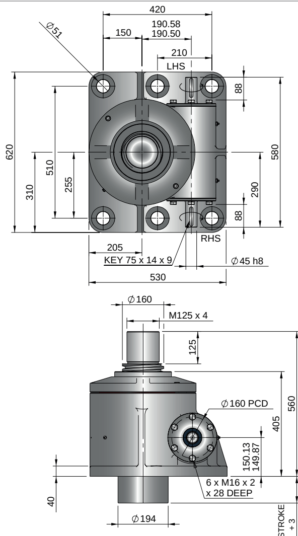
Upright EMT1000-V00
